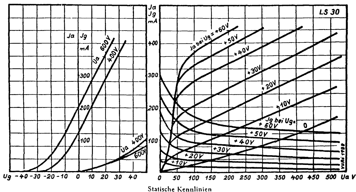
Statische Kennlinien
