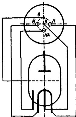
Anschlußskizze
