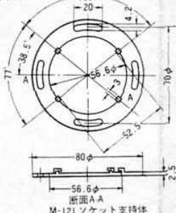
M-121 ソケット支持体
