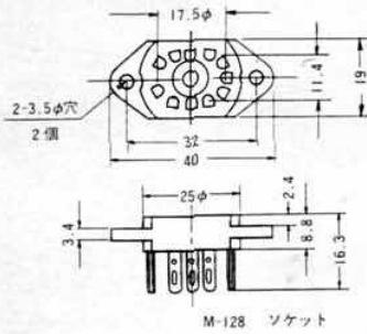
M-128 ソケット
