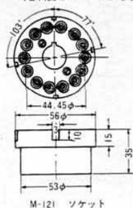
M-121 ソケット
