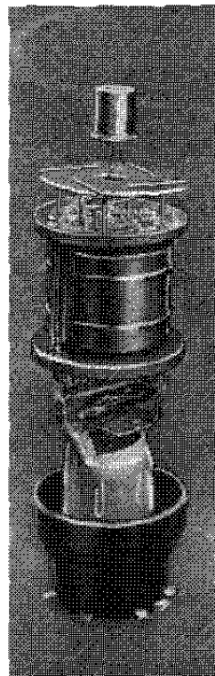
Construction intérieure de l'octode changeuse de fréquence KK 2.
