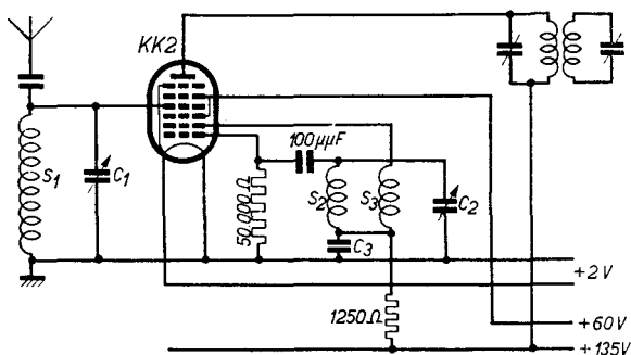
Schaltungsbeispiel ohne Patentobligo unsererseits. Prinzipialschaltung für die Verwendung der KK2 auf Kurzwellen.
