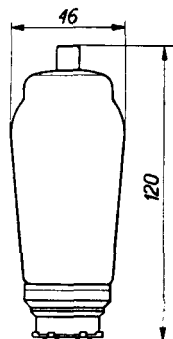
Abmessungen.
