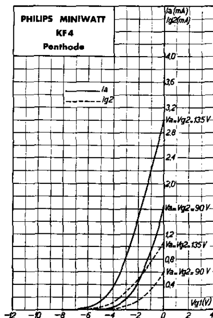
Courant d'anode et courant de grille-écran en fonction de la tension négative de la grille de commande V_a = V_{g2} = 135 V et V_a = V_{g2} = 90 V.
