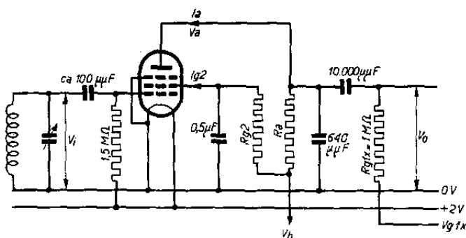
Montage du tube KF 4 comme détectrice grille avec couplage par résistance sans réaction.
