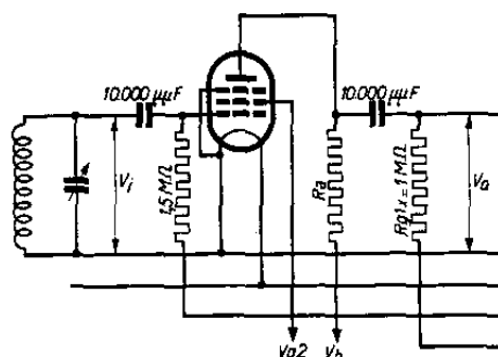
Montage du tube KF 4 comme détectrice plaque avec couplage par résistance.
