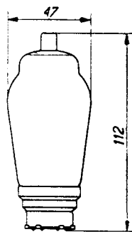
Abmessungen.
