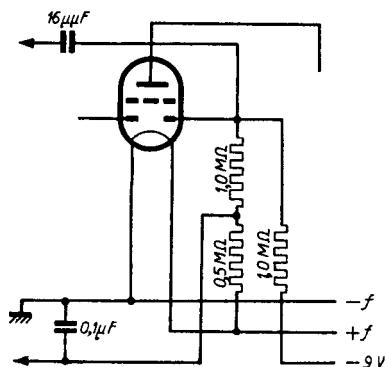
Schaltung ohne Patentobliga- unsererseits.
