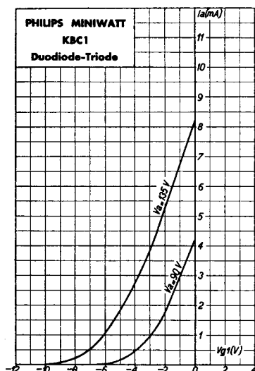
I_a/V_{g1} -Kurven des Triodenteiles der Röhre KBC 1.
