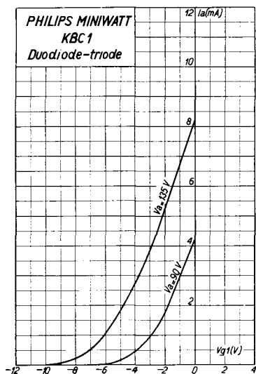
Abb. 8 I_a/V_g -Kennlinien der Röhre KBC 1.
