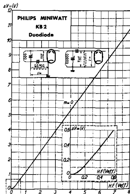
Accroissement de la tension continue ( \Delta V ) aux bornes de la résistance de fuite en fonction de la tension alternative à haute fréquence non modulée. Cette courbe s'applique au cas d'une résistance de fuite de 0,5 mégohm
