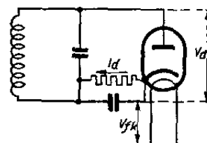
Principe du montage de la duodiode; définition de V_d et de I_d .
