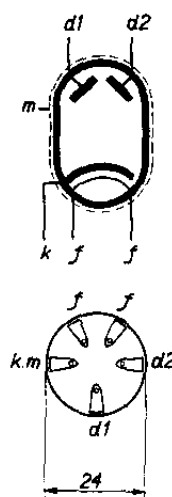
Disposition des électrodes et connexions du culot du tube KB 2.
