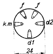
Elektroden- anschlüsse am Sockel.
