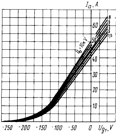
Усредненные анодно-сеточные характеристики: U_{g2} = 1500 \text{ В}; U_f = 18 \text{ В} Averaged Anode-Grid Characteristic Curves: U_f = 18 \text{ В}; U_{g2} = 1,500 \text{ В}
