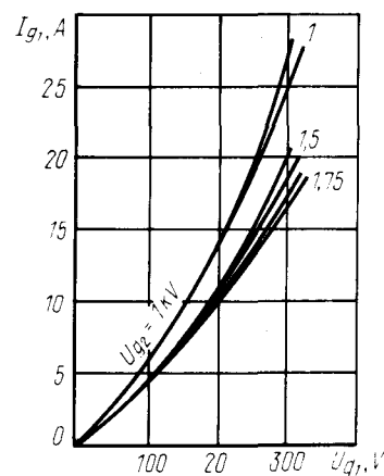
Сеточные характеристики: U_{g2} = 1000 \text{ В}; U_i = 18 \text{ В} Grid Characteristic Curves: U_i = 18 \text{ В}; U_a = 1-8 \text{ кВ}
