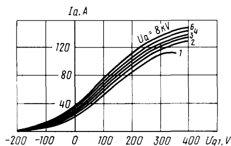
Анодно-сеточные характеристики: U_{g2} = 1000 \text{ В}; U_i = 18 \text{ В} Anode-Grid Characteristic Curves: U_i = 18 \text{ В}; U_{g2} = 1,000 \text{ В}
