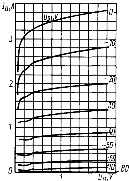
Усредненные анодные характеристики: U_i = 12,6 В; U_{g2} = 350 В
