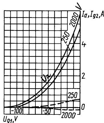
Усредненные анодно-сеточные и сеточные характеристики: U_1 = 27 \text{ В}; U_{g2} = 400 \text{ В}; — ток анода ( I_a ); --- ток сетки второй ( I_{g2} ) Averaged Anode-Grid and Grid Characteristic Curves: U_1 = 27 \text{ В}; U_{g2} = 400 \text{ В}; — I_a ; --- I_{g2}
