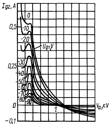
Усредненные сеточно-анодные характеристики: U_1 = 27 \text{ В}; U_{g2} = 400 \text{ В} Averaged Grid-Anode Characteristic Curves: U_1 = 27 \text{ V}; U_{g2} = 400 \text{ V}
