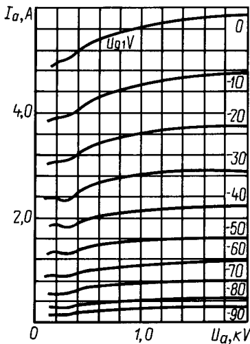
Усредненные анодные характеристики: U_1 = 27 \text{ В}; U_{g2} = 400 \text{ В} Averaged Anode Characteristic Curves: U_1 = 27 \text{ V}; U_{g2} = 400 \text{ V}
