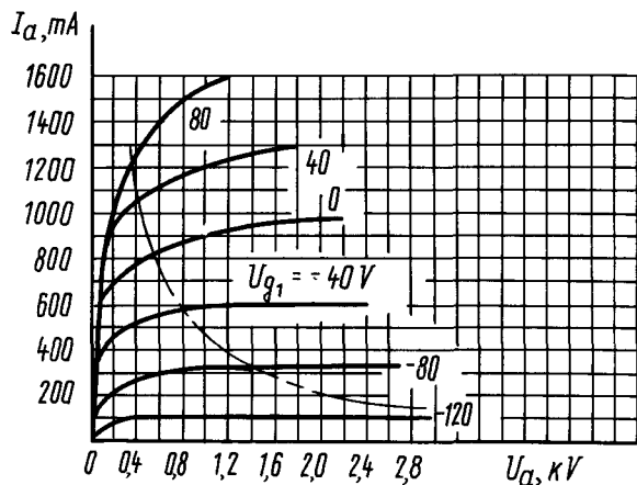
Усредненные анодные характеристики: U_i = 12.6 \text{ В} ; U_{g2} = 0.5 \text{ кВ} ; — — — наибольшая мощность, рассеиваемая анодом ( P_{a \max} ) Averaged Anode Characteristic Curves: U_i = 12.6 \text{ V} ; U_{g2} = 0.5 \text{ кВ} ; — — — ( P_{a \max} )
