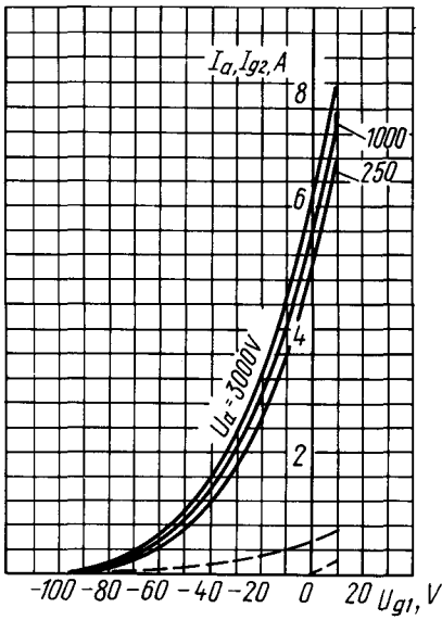
Усредненные характеристики: U_i = 27\text{ В}; U_{g2} = 300\text{ В}; — — — — — анодно-сеточные; — — — — — сеточные (по сетке второй); — — — — — сеточные (по сетке первой) Averaged Characteristic Curves: U_i = 27\text{ В}; U_{g2} = 300\text{ В}; — — — — — anode grid; — — — — — grid 2; — — — — — grid 1
