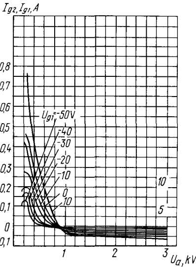
Усредненные сеточно-анодные характеристики: U_i = 27\text{ В}; U_{g2} = 300\text{ В}; — — — — — ток сетки второй; — — — — — ток сетки первой Averaged Grid-Anode Characteristic Curves: U_i = 27\text{ В}; U_{g2} = 300\text{ В}; — — — — — I_{g2}; — — — — — I_{g1}
