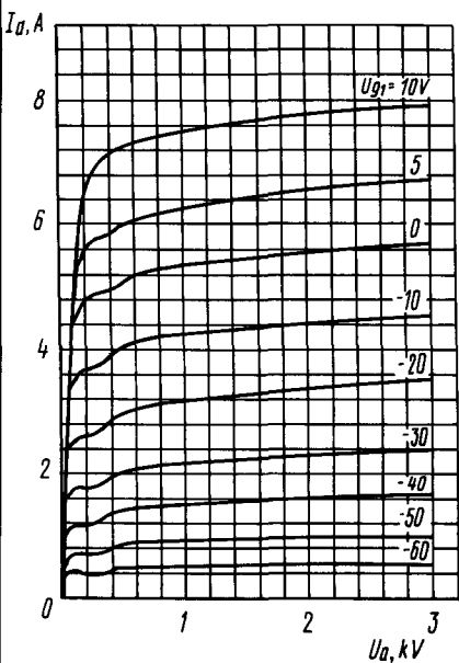
Усредненные анодные характеристики: U_i = 27\text{ В}; U_{g2} = 300\text{ В} Averaged Anode Characteristic Curves: U_i = 27\text{ V}; U_{g2} = 300\text{ V}
