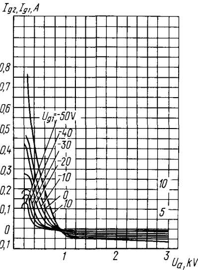
Усредненные сеточно-анодные характеристики: U_i = 27\text{ В} ; U_{g2} = 300\text{ В} ; — — — — — ток сетки второй; — — — — — ток сетки первой Averaged Grid-Anode Characteristic Curves: U_i = 27\text{ В} ; U_{g2} = 300\text{ В} ; — — — — — I_{g2} ; — — — — — I_{g1}
