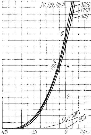
Усредненные сеточные и анодно-сеточные характеристики: U_i = 27\text{ В}; U_{g2} = 300\text{ В}; — — — — — анодные; — — — — — сеточные по второй сетке; — · — — — сеточные по первой сетке Averaged Grid and Anode-Grid Characteristic Curves: U_i = 27\text{ В}; U_{g2} = 300\text{ В}; — — — — — anode; — — — — — grid 2; — · — — — grid 1
