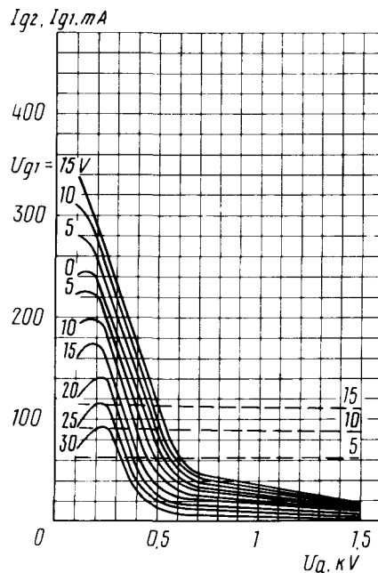
Усредненные сеточно-анодные характеристики: U_f = 26 \text{ B} ; U_{g2} = 400 \text{ B} ;
