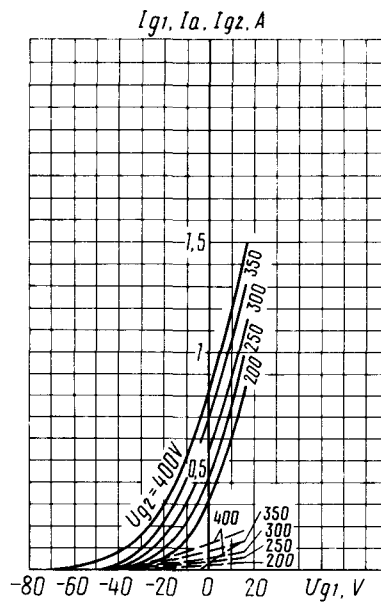
Усредненные анодно-сеточные и сеточные характеристики: U_f = 26 \text{ B} ; U_{g2} = 300 \text{ B} ;
