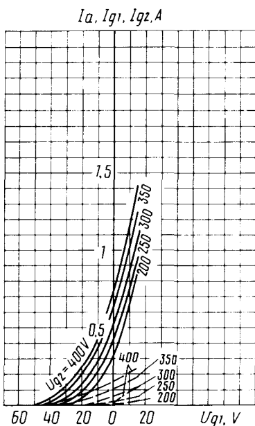
Усредненные анодно-сеточные и сеточные характеристики: U_f = 26 \text{ B} ; U_{g2} = 400 \text{ B} ;
