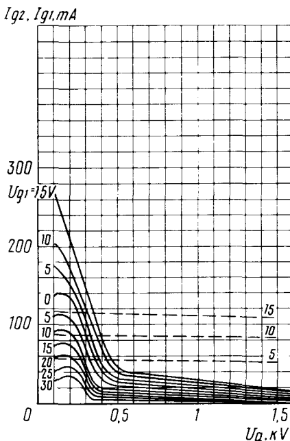
Усредненные сеточно-анодные характеристики: U_f = 26 \text{ B} ; U_{g2} = 300 \text{ B} ;
