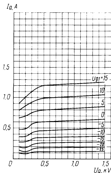
Усредненные анодные характеристики: U_f = 26 \text{ B} ; U_{g2} = 300 \text{ B}
