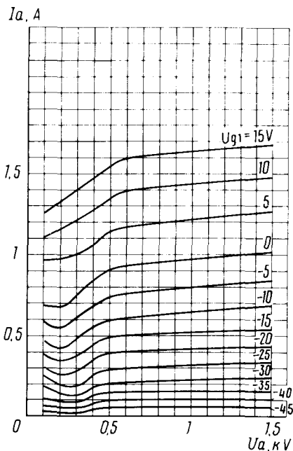
Усредненные анодные характеристики: U_f = 26 \text{ B} ; U_{g2} = 400 \text{ B}
