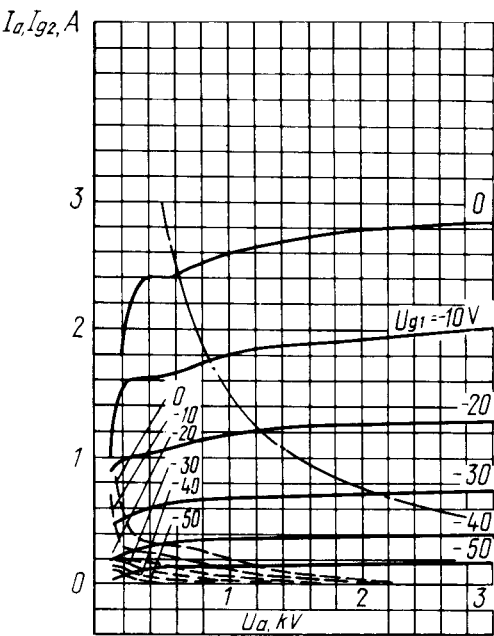
Усредненные характеристики: U_i = 12,6 \text{ В}; U_{g2} = 350 \text{ В}; U_{g3} = 0; — анодные; --- сеточно-анодные (по сетке второй); - · - наибольшая мощность, рассеиваемая анодом ( P_{a \text{ max}} )
