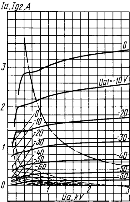
Усредненные характеристики: U_i = 12,6 \text{ В}; U_{g2} = 400 \text{ В}; U_{g3} = 0 \text{ В}; — анодные; --- сеточно-анодные (по сетке второй); - · - наибольшая мощность, рассеиваемая анодом ( P_{a \text{ max}} )
