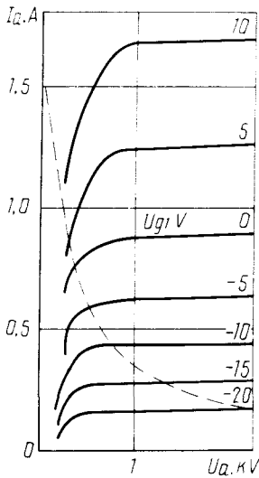
Усредненные анодные характеристики: U_i = 6\text{ В}; U_{g2} = 400\text{ В}; — · — наибольшая мощность, рассеиваемая анодом ( P_{a\text{ max}} ) Averaged Anode Characteristic Curves: U_i = 6\text{ В}; U_{g2} = 400\text{ В}; — · — P_{a\text{ max}}
