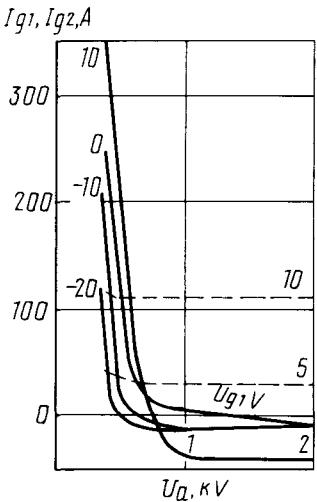
Усредненные характеристики: U_i = 6\text{ В}; U_{g2} = 400\text{ В}; — сеточно-анодные (по сетке второй); - - - сеточно-анодные (по сетке первой) Averaged Characteristic Curves: U_i = 6\text{ В}; U_{g2} = 400\text{ В}; — grid 2-anode; - - - grid 1-anode
