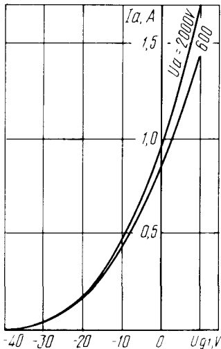
Усредненные анодно-сеточные характеристики: U_i = 6\text{ В}; U_{g2} = 400\text{ В} Averaged Anode-Grid Characteristic Curves: U_i = 6\text{ В}; U_{g2} = 400\text{ В}
