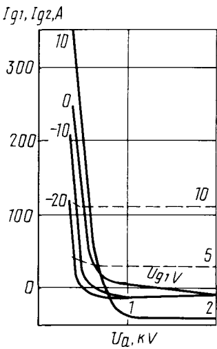
Усредненные характеристики: U_i = 6 \text{ В}; U_{g2} = 400 \text{ В}; — сеточно-анодные (по сетке второй); - - - сеточно-анодные (по сетке первой) Averaged Characteristic Curves: U_i = 6 \text{ В}; U_{g2} = 400 \text{ В}; — grid 2-anode; - - - grid 1-anode
