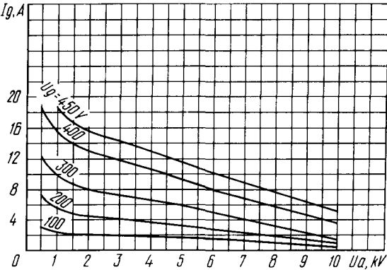
Усредненные сеточно-анодные характеристики: U_t = 13,5 \text{ В} Averaged Grid-Anode Characteristic Curves: U_t = 13.5 \text{ V}
