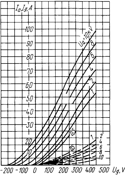
Усредненные характеристики: U_f = 13,5 \text{ В} ; — анодно-сеточные; --- сеточные Averaged Characteristic Curves: U_f = 13.5 \text{ V} ; — anode-grid; --- grid
