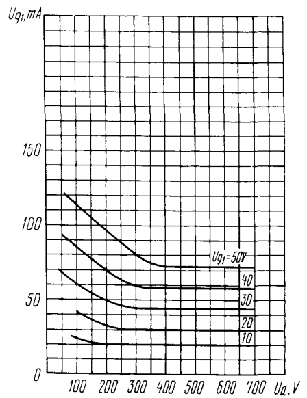
Усредненные сеточно-анодные характеристики (для одного тетрода): U_i = 6,3 \text{ В}; U_{g2} = 300 \text{ В}
