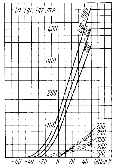
Усредненные анодно-сеточные и сеточные харак- теристики (для одного тетрода): U_i = 6,3 \text{ В}; U_a = 700 \text{ В};
