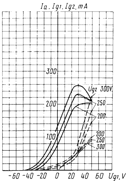
Усредненные анодно-сеточные характеристики (для одного тетрода): U_i = 6,3 \text{ В}; U_{g2} = 200 \text{ В};
