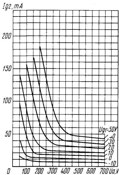
Усредненные сеточно-анодные характеристики (для одного тетрода): U_i = 6,3 \text{ В}; U_{g2} = 300 \text{ В}
