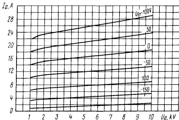
Усредненные анодные характеристики: U_f = 8,3 \text{ В} ; U_{g2} = 1,5 \text{ кВ} Averaged Anode Characteristic Curves: U_f = 8,3 \text{ В} ; U_{g2} = 1,5 \text{ кВ}
