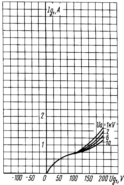
Усредненные сеточные характеристики (по сетке первой): U_i = 8,3 \text{ В}; U_{g2} = 1 \text{ кВ} Averaged Grid 1 Characteristic Curves: U_i = 8.3 \text{ V}; U_{g2} = 1 \text{ kV}
