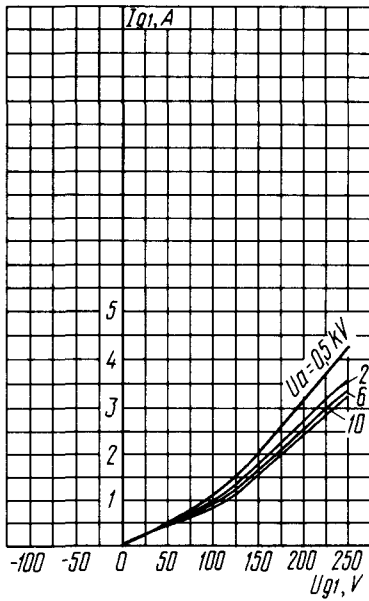
Усредненные сеточные характеристики (по сетке первой): U_i = 8,3 \text{ В}; U_{g2} = 500 \text{ В} Averaged Grid 1 Characteristic Curves: U_i = 8.3 \text{ V}; U_{g2} = 500 \text{ V}
