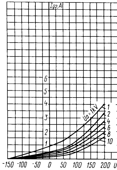
Усредненные сеточные характеристики (по сетке второй): U_i = 8,3 \text{ В}; U_{g2} = 1 \text{ кВ} Averaged Grid 2 Characteristic Curves: U_i = 8.3 \text{ V}; U_{g2} = 1 \text{ kV}
