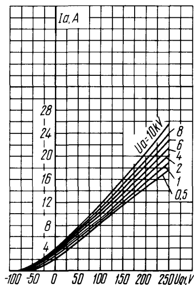
Усредненные анодно-сеточные характеристики: U_1 = 8,3 \text{ В}; U_{g2} = 500 \text{ В}
