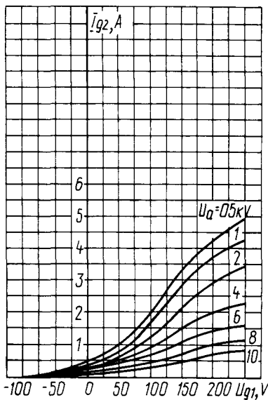
Усредненные сеточные характеристики (по сетке второй): U_i = 8,3 \text{ В}; U_{g2} = 500 \text{ В} Averaged Grid 2 Characteristic Curves: U_i = 8.3 \text{ V}; U_{g2} = 500 \text{ V}
