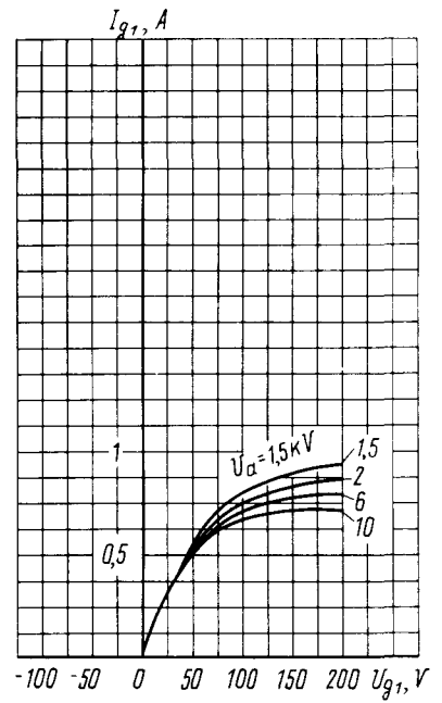
Усредненные сеточные характеристики (по сетке первой): U_i = 8,3 \text{ В}; U_{g2} = 1,5 \text{ кВ} Averaged Grid 1 Characteristic Curves: U_i = 8.3 \text{ V}; U_{g2} = 1.5 \text{ kV}
