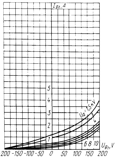
Усредненные сеточные характеристики (по сетке второй): U_i = 8,3 \text{ В}; U_{g2} = 1,5 \text{ кВ} Averaged Grid 2 Characteristic Curves: U_i = 8.3 \text{ V}; U_{g2} = 1.5 \text{ kV}
