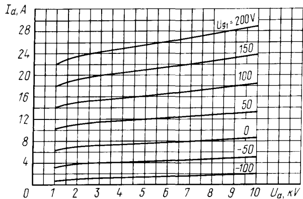
Усредненные анодные характеристики: U_f = 8,3 \text{ В} ; U_{g2} = 1 \text{ кВ} Averaged Anode Characteristic Curves: U_f = 8,3 \text{ В} ; U_{g2} = 1 \text{ кВ}
