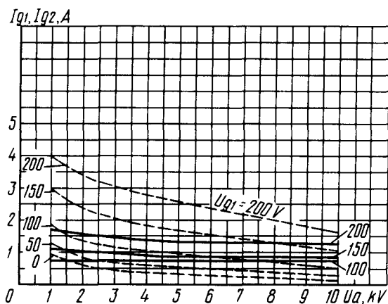
Усредненные характеристики: U_1 = 8,3 \text{ В}; U_{g2} = 1 \text{ кВ}; — сеточно-анодные (по сетке первой); --- сеточно-анодные (по сетке второй)
