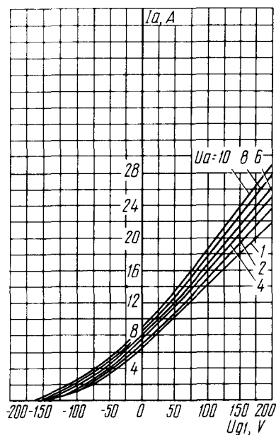
Усредненные анодно-сеточные характеристики: U_1 = 8,3 \text{ В}; U_{g2} = 1,5 \text{ кВ}
