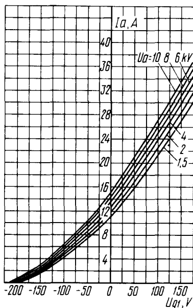
Усредненные анодно-сеточные характеристики: U_1 = 8,3 \text{ В}; U_{g2} = 1 \text{ кВ}
