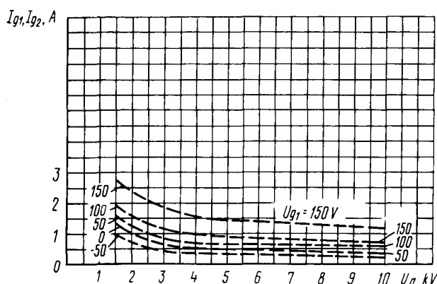
Усредненные характеристики: U_1 = 8,3 \text{ В}; U_{g2} = 1,5 \text{ кВ}; — сеточно-анодные (по сетке первой); --- сеточно-анодные (по сетке второй)
