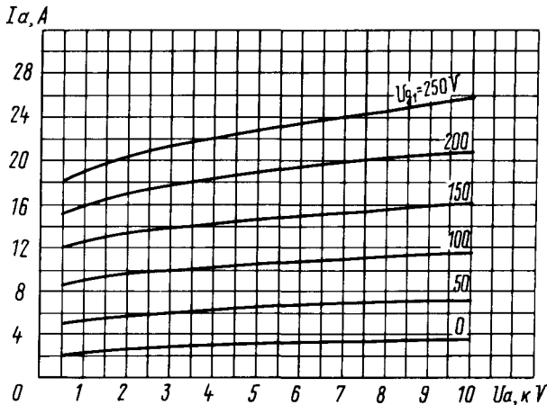
Усредненные анодные характеристики: U_f = 8,3 \text{ В} ; U_{g2} = 500 \text{ В} Averaged Characteristic Curves: U_f = 8,3 \text{ В} ; U_{g2} = 500 \text{ В}
