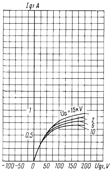
Усредненные сеточные характеристики (по сетке первой): U_i = 8,3 \text{ В}; U_{g2} = 1,5 \text{ кВ} Averaged Grid 1 Characteristic Curves: U_i = 8.3 \text{ В}; U_{g2} = 1.5 \text{ кВ}
