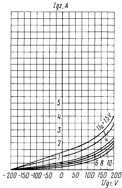
Усредненные сеточные характеристики (по сетке второй): U_i = 8,3 \text{ В}; U_{g2} = 1,5 \text{ кВ} Averaged Grid 2 Characteristic Curves: U_i = 8.3 \text{ В}; U_{g2} = 1.5 \text{ кВ}
