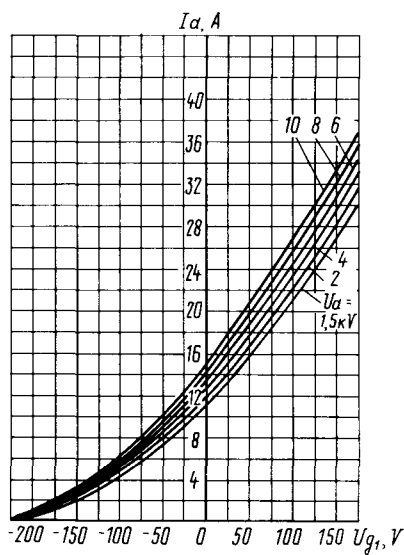
Усредненные анодно-сеточные характеристики: U_i = 8,3 \text{ В}; U_{g2} = 1,5 \text{ кВ} Averaged Anode-Grid Characteristic Curves: U_i = 8.3 \text{ V}; U_{g2} = 1.5 \text{ kV}
