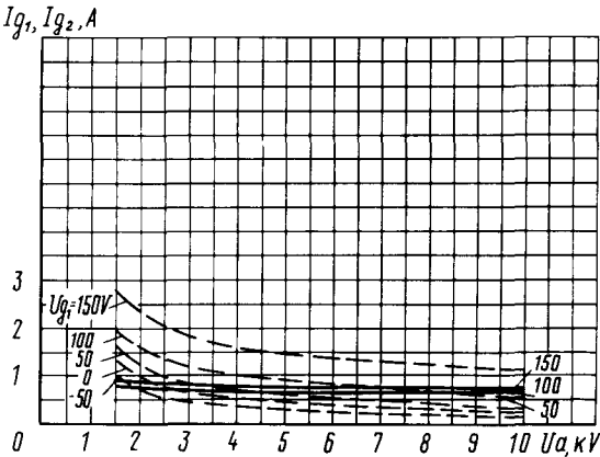
Усредненные характеристики: U_f = 8,3 \text{ В} ; U_{g2} = 1,5 \text{ кВ} ; — сеточно-анодные (по сетке первой); --- сеточно-анодные (по сетке второй) Averaged Characteristic Curves: U_f = 8.3 \text{ V} ; U_{g2} = 1.5 \text{ kV} ; — grid 1-anode; --- grid 2-anode
