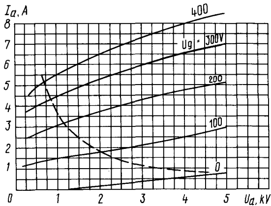
Усредненные анодные характеристики: U_i = 12.6\text{ В} ; - - - - - наибольшая мощность, рассеиваемая анодом ( P_{a, max} ) Averaged Anode Characteristic Curve: U_i = 12.6\text{ V} ; - - - - - P_{a, max}
