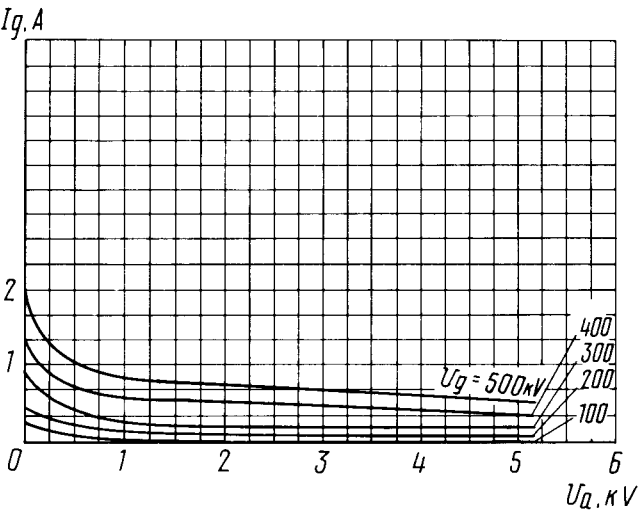
Усредненные сеточно-анодные характеристики: U_f = 6,3 \text{ В} Averaged Grid-Anode Characteristic Curves: U_f = 6.3 \text{ V}
