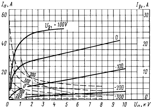
Усредненные характеристики: U_i = 14 В; U_{g2} = 1,75 кВ; — — — анодные; — — — сеточно-анодные; — · — наибольшая допустимая мощность, рассеиваемая анодом ( P_{a \max} )
