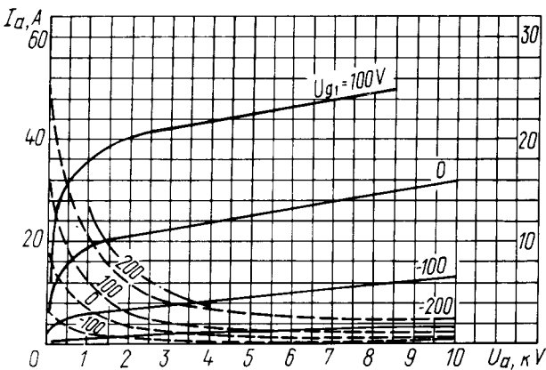
Усредненные характеристики: U_i = 14 В; U_{g2} = 1,5 кВ; — — — анодные; — — — сеточно-анодные; — · — наибольшая допустимая мощность, рассеиваемая анодом ( P_{a \max} )
