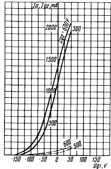
Усредненные характеристики: U_1 = 8,3 \text{ В}; U_a = 1 \text{ кВ}; U_{q3} = 0 \text{ В}; — анодные; - - - сеточные Averaged Characteristic Curves: U_1 = 8.3 \text{ В}; U_{a2} = 1 \text{ кВ}; U_{q3} = 0; — anode; - - - grid
