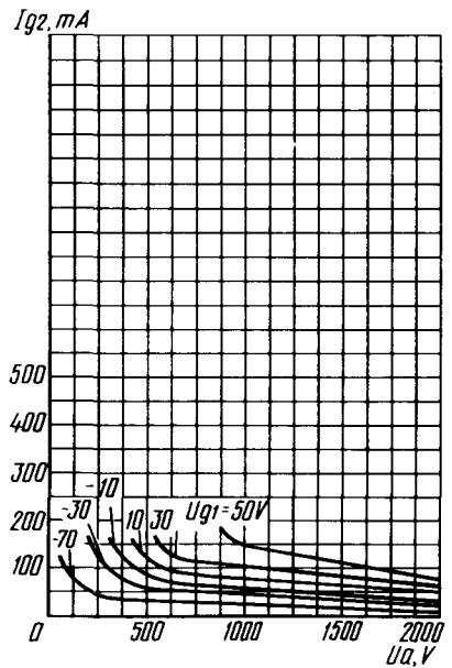
Усредненные сеточно-анодные характеристики (по сетке второй): U_1 = 8,3 \text{ В}; U_{q2} = 0,6 \text{ кВ}; U_{q3} = 0 \text{ В} Averaged Grid 2-Anode Characteristic Curves: U_1 = 8.3 \text{ V}; U_{q2} = 0.6 \text{ кВ}; U_{q3} = 0
