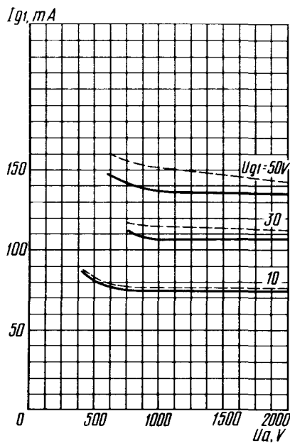
Усредненные сеточно-анодные характеристики (по сетке первой): U_1 = 8,3 \text{ В}; U_{q3} = 0 \text{ В}; — U_{q2} = 0,6 \text{ кВ}; - - - U_{q2} = 0,5 \text{ кВ} Averaged Grid 1-Anode Characteristic Curves: U_1 = 8.3 \text{ В}; U_{q3} = 0; — at U_{q2} = 0.6 \text{ кВ}; - - - at U_{q2} = 0.5 \text{ кВ}
