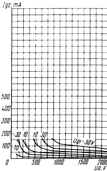
Усредненные сеточно-анодные характеристики (по сетке второй): U_1 = 8,3 \text{ В}; U_{q2} = 0,5 \text{ кВ}; U_{q3} = 0 \text{ В} Averaged Grid 2-Anode Characteristic Curves: U_1 = 8.3 \text{ V}; U_{q2} = 0.5 \text{ кВ}; U_{q3} = 0
