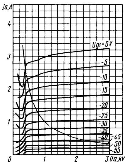
Усредненные анодные характеристики: U_1 = 12,6 \text{ В} ; U_2 = 350 \text{ В} ; — — — наибольшая мощность, рассеиваемая анодом ( P_{a \text{ max}} ) Averaged Anode Characteristic Curves: U_1 = 12.6 \text{ V} ; U_2 = 350 \text{ V} ; — — — P_{a \text{ max}}
