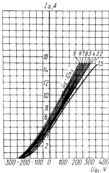
Усредненные анодно-сеточные характеристики: U_i = 6,3 \text{ В}; U_{g2} = 1,5 \text{ кВ}
