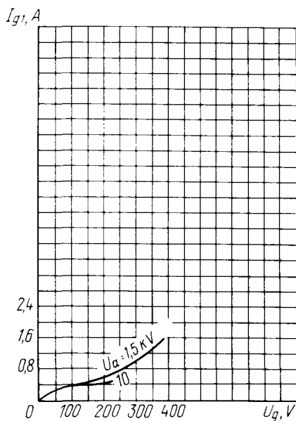
Усредненные сеточные характеристики (по сетке второй): U_i = 6,3 \text{ В}; U_{g2} = 1,5 \text{ кВ}
