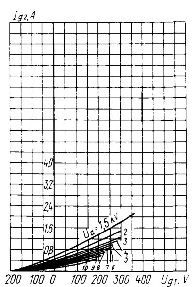
Усредненные сеточные характеристики (по сетке второй): U_i = 6,3 \text{ В}; U_{g2} = 1,5 \text{ кВ}
