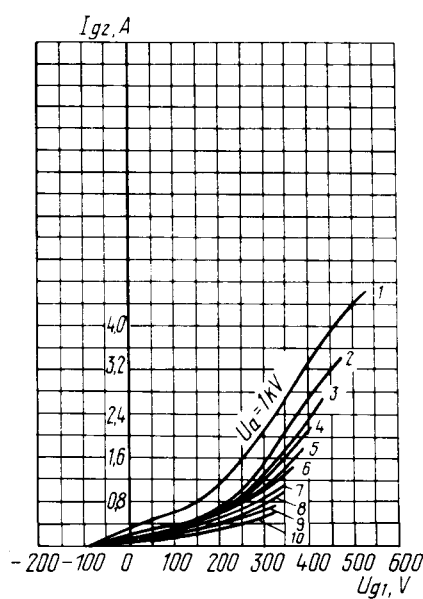
Усредненные сеточные характеристики (по сетке второй): U_i = 6,3 \text{ В}; U_{g2} = 1 \text{ кВ}
