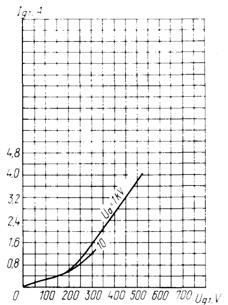
Усредненные сеточные характеристики (по сетке первой): U_i = 6,3 \text{ В}; U_{g2} = 1 \text{ кВ}
