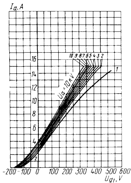
Усредненные анодно-сеточные характеристики: U_i = 6,3 \text{ В}; U_{g2} = 1,5 \text{ кВ}
