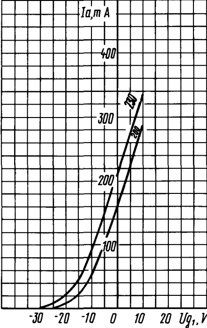
Усредненные анодно-сеточные характеристики (каждого тетрода): U_i = 12.6\text{ V} ; U_a = 550\text{ V} Averaged Anode-Grid Characteristic Curves (Each Tetrode): U_i = 12.6\text{ V} ; U_a = 550\text{ V}
