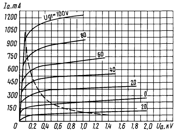
Усредненные анодные характеристики: U_f = 10 \text{ В} ; U_{g2} = 0.4 \text{ кВ} ; — — — наибольшая мощность, рассеиваемая анодом ( P_{a \text{ max}} ); напряжение лучеобразующих пластин ( U_{лп} ) равно 0 В Averaged Anode Characteristic Curves: U_f = 10 \text{ V} ; U_{g2} = 0.4 \text{ kV} ; — — — P_{a \text{ max}} beam-forming plates voltage U_{лп} is 0
