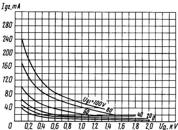
Усредненные сеточно-анодные характеристики (по сетке второй): U_f = 10 \text{ В} ; U_{g2} = 0.3 \text{ кВ} ; напряжение лучеобразующих пластин ( U_{лп} ) равно 0 В Averaged Grid 2-Anode Characteristic Curves: U_f = 10 \text{ V} ; U_{g2} = 0.3 \text{ kV} ; beam-forming plates voltage U_{лп} is 0
