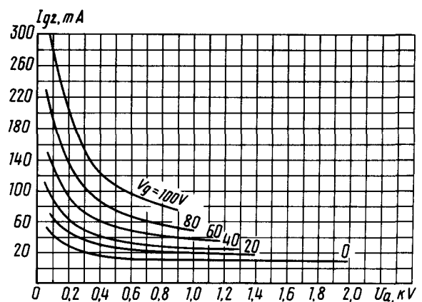
Усредненные сеточно-анодные характеристики (по сетке второй): U_f = 10 \text{ В} ; U_{g2} = 0.4 \text{ кВ} ; напряжение лучеобразующих пластин ( U_{лп} ) равно 0 В Averaged Grid 2-Anode Characteristic Curves: U_f = 10 \text{ V} ; U_{g2} = 0.4 \text{ kV} ; beam-forming plates voltage U_{лп} is 0
