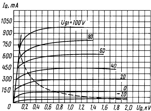
Усредненные анодные характеристики: U_f = 10 \text{ В} ; U_{g2} = 0.3 \text{ кВ} ; — — — наибольшая мощность, рассеиваемая анодом ( P_{a \text{ max}} ); напряжение лучеобразующих пластин ( U_{лп} ) равно 0 В Averaged Anode Characteristic Curves: U_f = 10 \text{ V} ; U_{g2} = 0.3 \text{ kV} ; — — — P_{a \text{ max}} beam-forming plates voltage U_{лп} is 0
