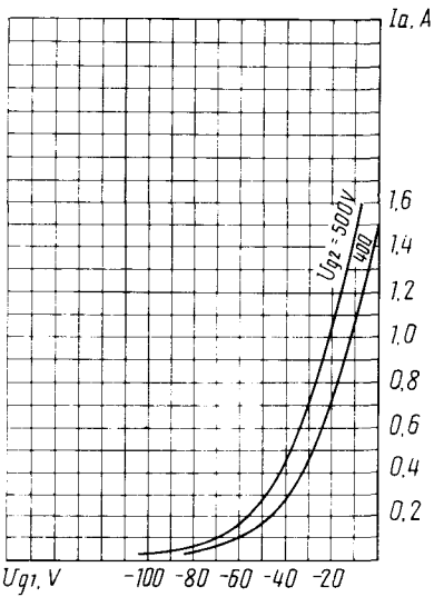
Усредненные анодно-сеточные характеристики: U_i = 26\text{ В}; U_a = 2\text{ кВ} Averaged Anode-Grid Characteristic Curves: U_i = 26\text{ V}; U_a = 2\text{ кВ}
