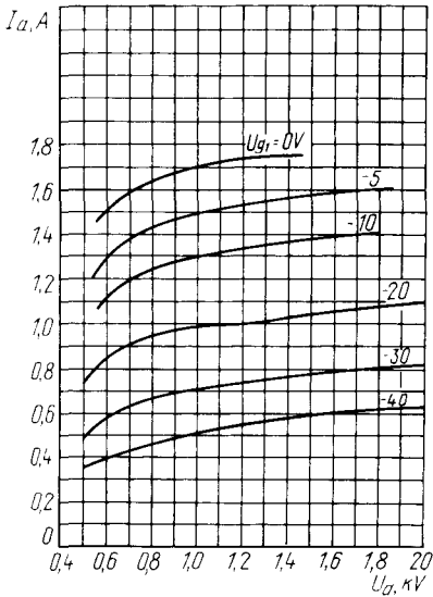
Усредненные анодные характеристики: U_i = 26\text{ В}; U_{g2} = 500\text{ В} Averaged Anode Characteristic Curves: U_i = 26\text{ V}; U_{g2} = 500\text{ V}
