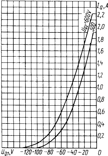
Усредненные анодно-сеточные характеристики: U_i = 26 \text{ В}; U_a = 2,5 \text{ кВ} Averaged Anode-Grid Characteristic Curves: U_i = 26 \text{ V}; U_a = 2.5 \text{ kV}
