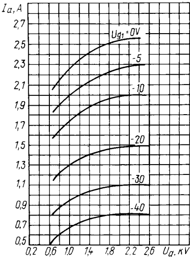
Усредненные анодные характеристики: U_i = 26 \text{ В}; U_{g2} = 600 \text{ В} Averaged Anode Characteristic Curves: U_i = 26 \text{ V}; U_{g2} = 600 \text{ V}
