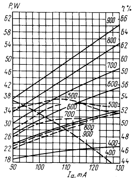
Усредненные характеристики в режиме автогенерации: U_i = 6,3 \text{ В} ; \lambda = 30 \text{ см} ; — колебательная мощность (P); --- коэффициент полезного действия ( \eta ) Averaged Characteristic Curves for Oscillation Mode: U_i = 6.3 \text{ V} ; \lambda = 30 \text{ cm} ; — oscillator output power (P); --- efficiency ( \eta )
