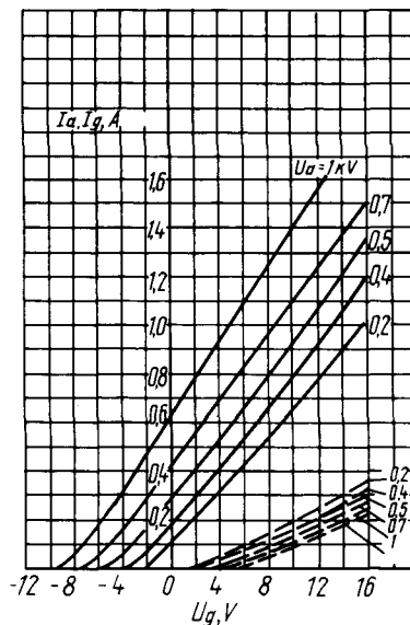
Усредненные анодно-сеточные и сеточные характеристики: U_i = 6,3 \text{ В} ; — анодно-сеточные; --- сеточные Averaged Anode-Grid and Grid Characteristic Curves: U_i = 6.3 \text{ V} ; — anode-grid; --- grid
