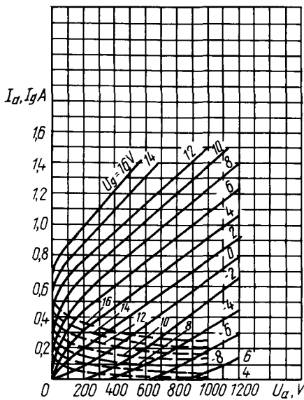
Усредненные анодно-сеточные характеристики: U_i = 6,3 \text{ В} ; — анодные; --- анодно-сеточные Averaged Anode-Grid Characteristic Curves: U_i = 6.3 \text{ V} ; — anode; --- anode-grid
