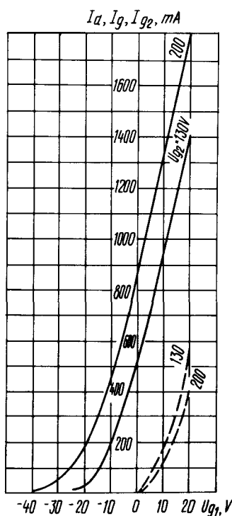
Усредненные анодно-сеточные и сеточные характеристики: U_f = 12,6 В; U_a = 1000 В; — ток анода ( I_a ); --- ток сетки первой ( I_{g1} ); ..... ток сетки второй ( I_{g2} )
