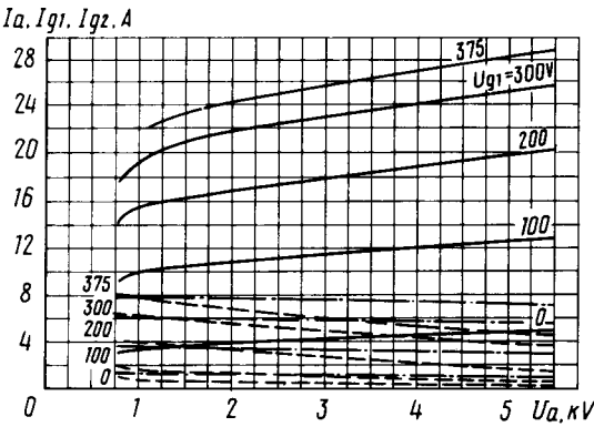
Усредненные характеристики: U_f = 3,4 В; U_{g2} = 0,8 кВ; — — — анодные; — — — сеточно-анодные (по сетке второй); — · — сеточно-анодные (по сетке первой) Averaged Characteristic Curves: U_f = 3.4 V; U_{g2} = 0.8 kV; — — — anode; — — — grid 2-anode; — · — grid 1-anode
