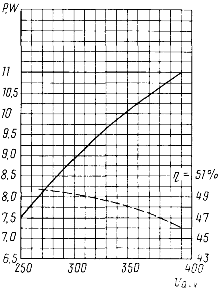
Усредненные характеристики: U_i = 6,3\text{ В} ; I_a = 60\text{ мА} ; \lambda = 50\text{ см} — — — — — колебательная мощность (P); — — — — — коэффициент полезного действия ( \eta ) Averaged Characteristic Curves: U_i = 6.3\text{ V} ; I_a = 60\text{ mA} ; \lambda = 50\text{ cm} — — — — — oscillator output power (P); — — — — — efficiency \eta
