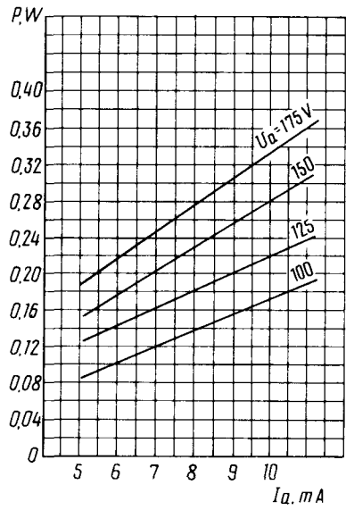
Усредненные характеристики зависимости колебательной мощности от тока анода: U_i = 6,3 \text{ В} Averaged Characteristic Curves Showing Oscillator Output Power versus Anode Current: U_i = 6.3 \text{ V}
