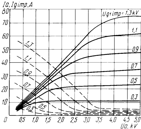
Усредненные характеристики: U_i = 26 В; отрицательное напряжение сетки ( U_g ) равно 200 В; — анодные; - - - сеточно-анодные Averaged Characteristic Curves: U_i = 26 V; negative grid voltage — 200 V; — anode; - - - grid-anode
