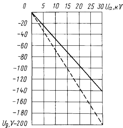
Усредненные характеристики зависимости отрицательного напряжения сетки от напряжения анода: U_i = 26 В; — напряжение запирания ( U_{g\text{cutoff}} ); - - - рекомендуемое напряжение смещения ( U_{gb} ) Averaged Characteristic Curves Showing Negative U_i = 26 V; — cutoff voltage U_{g\text{cutoff}} ; - - - recommended bias voltage U_{gb}
