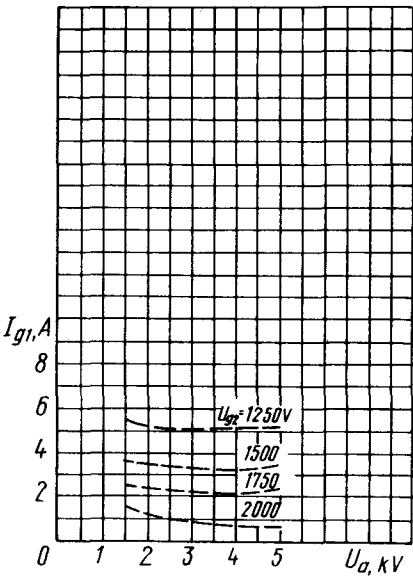
Усредненные сеточно-анодные характеристики (по сетке второй): избыточное напряжение сетки первой ( U_{g1} ) в импульсе равно 125 В Averaged Grid 2-Anode Characteristic Curves (at peak grid 1 excess voltage U_{g1 \text{ imp}} = 125 \text{ V} )
