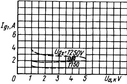
Усредненные сеточно-анодные характеристики (по сетке второй): избыточное напряжение сетки первой ( U_{g1} ) в импульсе равно 100 В Averaged Grid 2-Anode Characteristic Curves (at peak grid 1 excess voltage U_{g1 \text{ imp}} = 100 \text{ V} )
