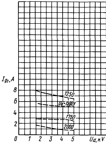
Усредненные сеточно-анодные характеристики (по сетке второй): избыточное напряжение сетки первой ( U_{g1} ) в импульсе равно 150 В Averaged Grid 2-Anode Characteristic Curves (at peak grid 1 excess voltage U_{g1 \text{ imp}} = 150 \text{ V} )
