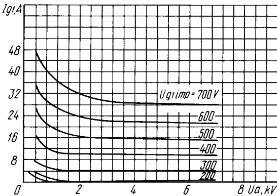
Усредненные импульсные сеточно-анодные характеристики (по сетке первой): U_1 = 9,5 \text{ В} ; U_{g2} = 1 \text{ кВ} Averaged Peak Grid 1-Anode Characteristic Curves: U_1 = 9.5 \text{ V} ; U_{g2} = 1 \text{ kV}
