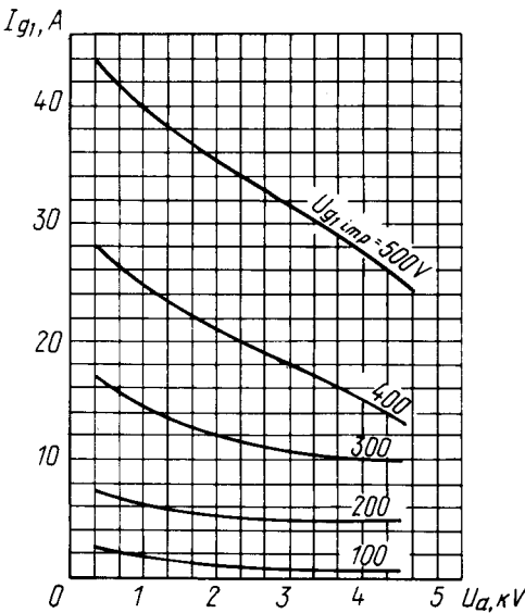
Усредненные импульсные сеточно-анодные характеристики (по сетке первой): U_1 = 9,5 \text{ В} ; U_{g2} = 400 \text{ В} Averaged Peak Grid 1-Anode Characteristic Curves: U_1 = 9.5 \text{ V} ; U_{g2} = 400 \text{ V}
