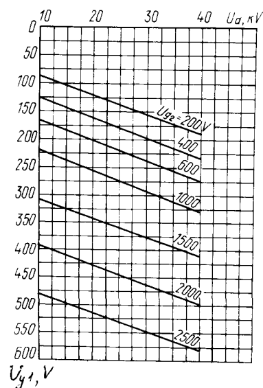
Усредненные характеристики зависимости напряжения записания сетки первой от напряжения анода: U_1 = 9,5 \text{ В} ; U_{g1} — напряжения записания
