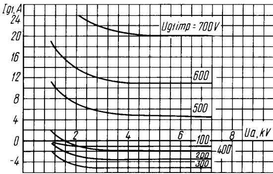
Усредненные импульсные сеточно-анодные характеристики (по сетке первой): U_1 = 9,5 \text{ В} ; U_{g2} = 2,5 \text{ кВ} Averaged Peak Grid 1-Anode Characteristic Curves: U_1 = 9.5 \text{ V} ; U_{g2} = 2.5 \text{ kV}
