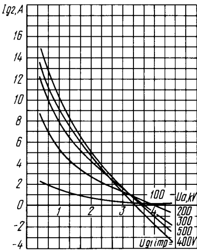
Усредненные импульсные сеточно-анодные характеристики (по сетке первой): U_1 = 9,5 \text{ В} ; U_{g2} = 400 \text{ В} Averaged Peak Grid 1-Anode Characteristic Curves: U_1 = 9.5 \text{ V} ; U_{g2} = 400 \text{ V}
