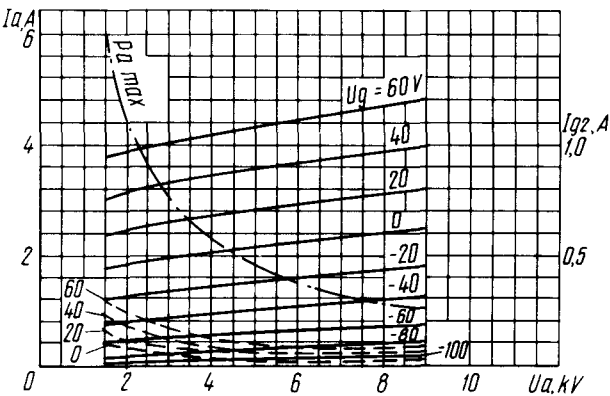
Усредненные характеристики: U_f = 5\text{ В} ; U_{g2} = 1\text{ кВ} ; — — — — — анодные; - - - - - сеточно-анодные; - · - · - · — — — — — наибольшая мощность, рассеиваемая анодом ( P_{a\text{ max}} ) Averaged Characteristic Curves: U_f = 5\text{ В} ; U_{g2} = 1\text{ кВ} ; — — — — — anode; - - - - - grid-anode; - · - · - · — — — — — P_{a\text{ max}}
