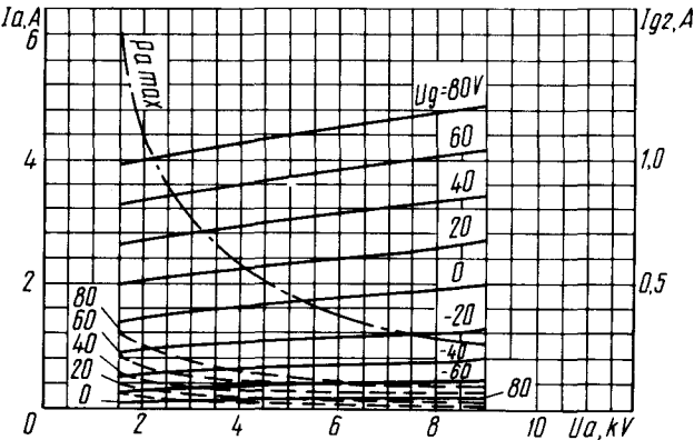
Усредненные характеристики: U_f = 5\text{ В} ; U_{g2} = 800\text{ В} ; — — — — — анодные; - - - - - сеточно-анодные; - · - · - · — — — — — наибольшая мощность, рассеиваемая анодом ( P_{a\text{ max}} ) Averaged Characteristic Curves: U_f = 5\text{ В} ; U_{g2} = 800\text{ В} ; — — — — — anode; - - - - - grid-anode; - · - · - · — — — — — P_{a\text{ max}}
