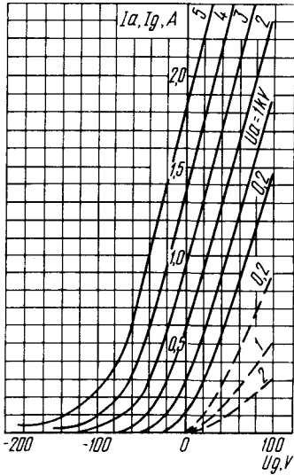
Усредненные характеристики: U_f = 6,3 \text{ В} ; — — — — — анодно-сеточные; сеточные Averaged Characteristic Curves: U_f = 6.3 \text{ V} ; — — — — — anode-grid; grid
