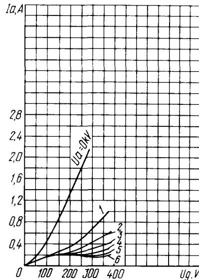
Усредненные анодно-сеточные характеристики: U_f = 10,5 \text{ В} Averaged Anode-Grid Characteristic Curves: U_f = 10.5 \text{ V}
