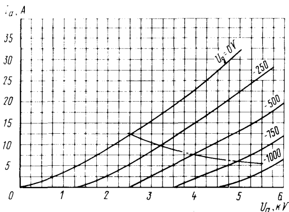
Усредненные анодно-сеточные характеристики: U_f = 10,5 \text{ В} Averaged Anode-Grid Characteristic Curves: U_f = 10.5 \text{ V}
