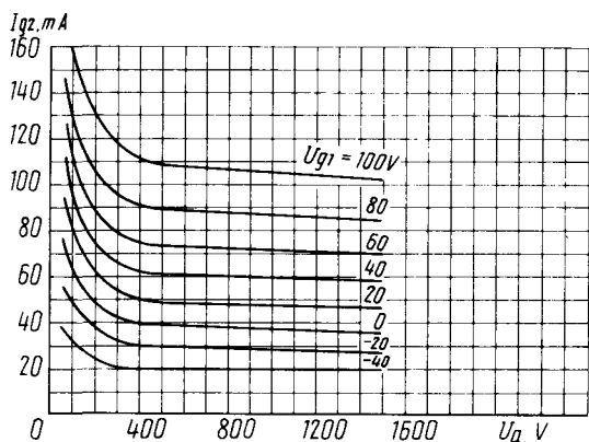
Усредненные сеточно-анодные характеристики (по сетке второй): U_1 = 20 \text{ В} ; U_{g2} = 0,4 \text{ кВ} ; U_{g3} = 50 \text{ В} Averaged Grid 2 Anode Characteristic Curves: U_1 = 20 \text{ В} ; U_{g2} = 0,4 \text{ кВ} ; U_{g3} = 50 \text{ В}
