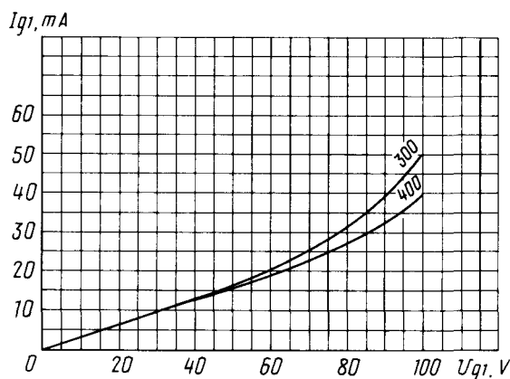
Усредненные сеточные характеристики: U_1 = 20 \text{ В} ; U_a = 1,5 \text{ кВ} ; U_{g3} = 50 \text{ В} Averaged Grid Characteristic Curves: U_1 = 20 \text{ В} ; U_a = 1,5 \text{ кВ} ; U_{g3} = 50 \text{ В}
