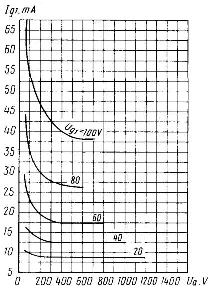
Усредненные сеточно-анодные характеристики: U_1 = 20 \text{ В} ; U_{g2} = 0,4 \text{ кВ} ; U_{g3} = 50 \text{ В} Averaged Grid-Anode Characteristic Curves: U_1 = 20 \text{ В} ; U_{g2} = 0,4 \text{ кВ} ; U_{g3} = 50 \text{ В}
