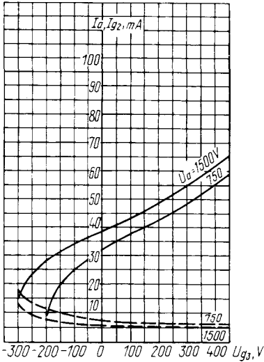
Усредненные характеристики: U_i = 20\text{ В}; U_{g2} = 0,3\text{ кВ}; U_{g1} = -50\text{ В}; — анодно-сеточные; --- сеточные (по сетке второй) Averaged Characteristic Curves: U_i = 20\text{ V}; U_{g2} = 0,3\text{ кВ}; U_{g1} = -50\text{ V}; — anode-grid; --- grid 2
